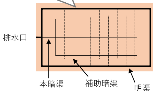
図1 明渠と補助暗渠の施工例
